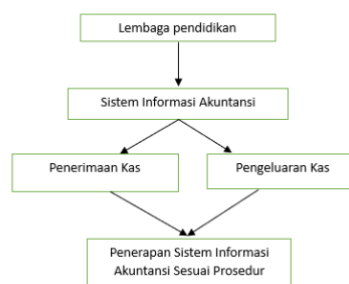
Gambar 1. Kerangka berpikir
